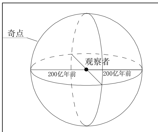
图 3: 观察者看到浩淼无垠的宇宙竟被奇点包裹着
