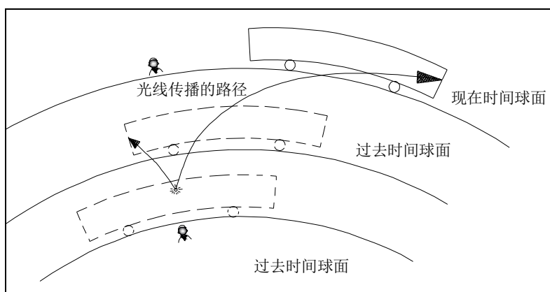
图 25: 地面上观察者看到的光线传播路径
