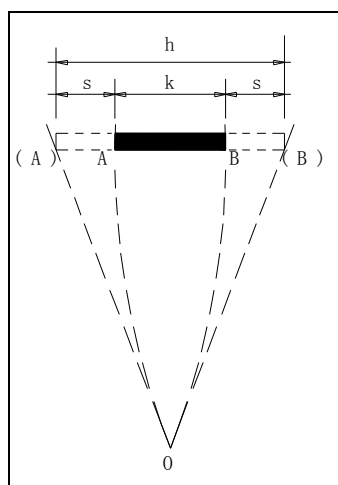
图 11: 观察尺度与实际尺度的偏差
