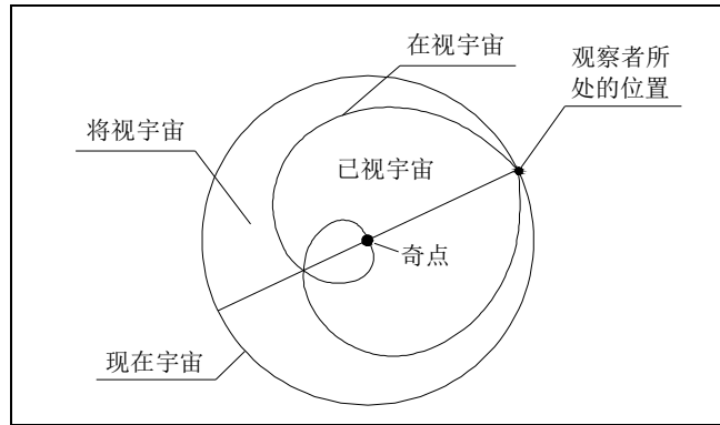
图 10: 视觉宇宙和时间球的对应关系
