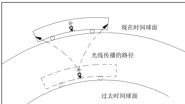
图 24: 车厢里观测者看到的光线传播路径
