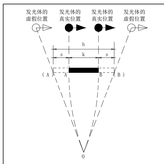
图 12: 实际观测时间比计算时间短
