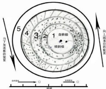
太阳构造 示意图
