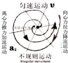
椭圆运动走势图
