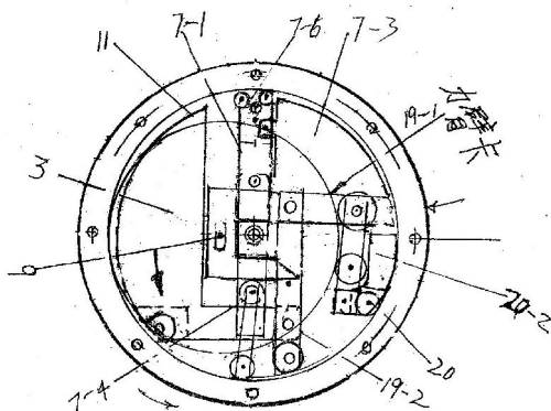
[001] 永动机两端部件做功示意图(二)
