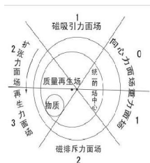
椭圆运动走势图
