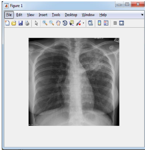
Fig. 7 Input image
